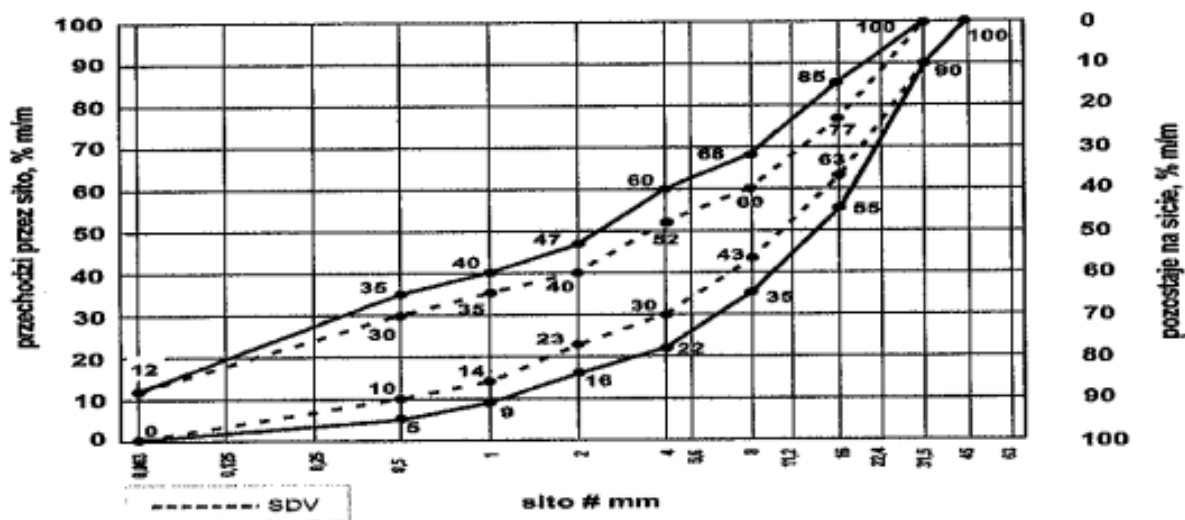
Rys.2 Uziarnienie mieszanki niezwiązanej odpowiednio 0/31,5 do podbudowy zasadniczej
