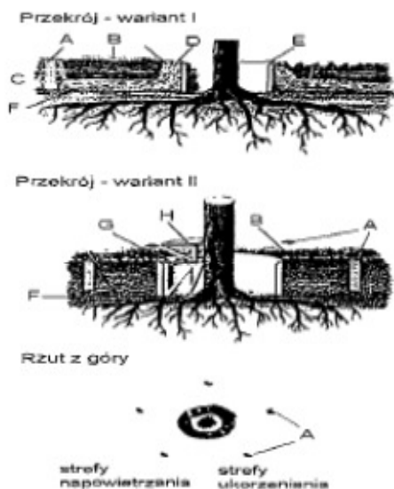
Rys. 5. Studzienka zabezpieczająca pień drzewa przy podwyższeniu terenu powyżej 0,5 m
